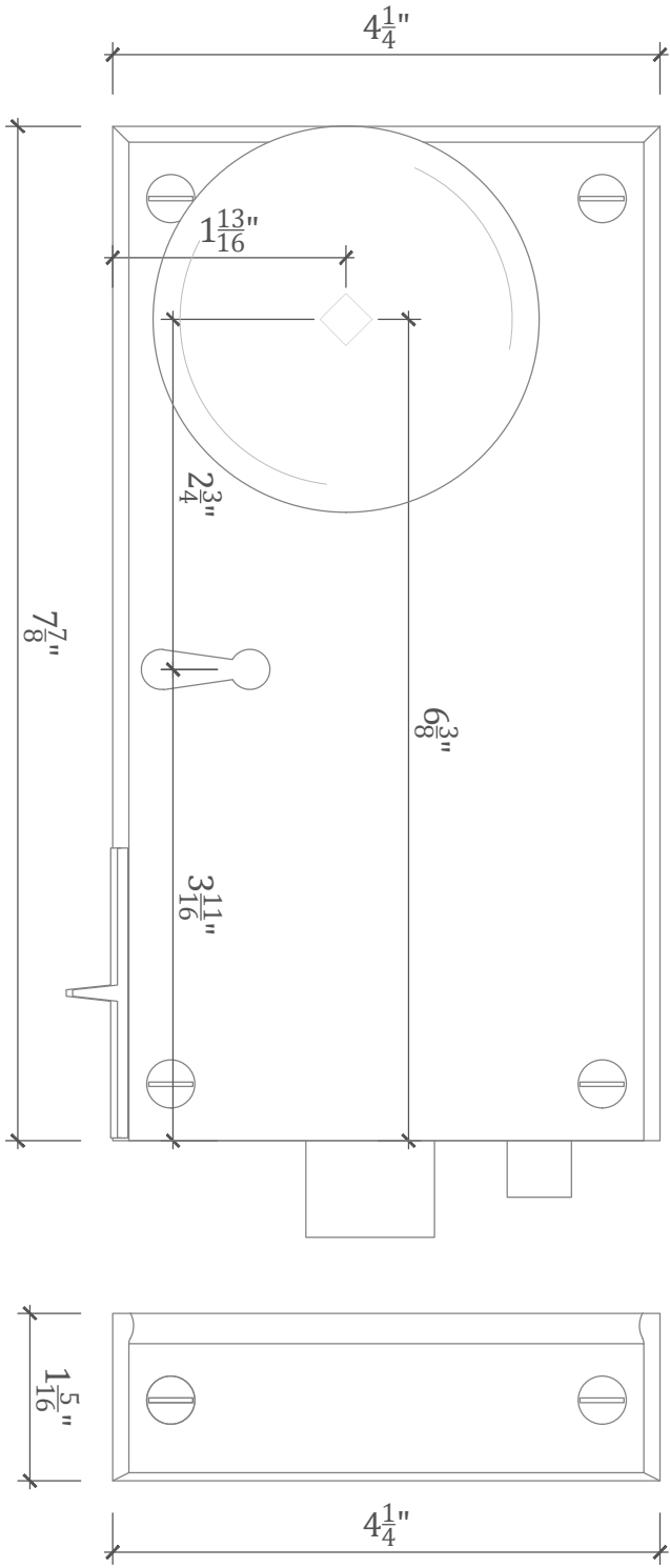
8" Rim Lock
